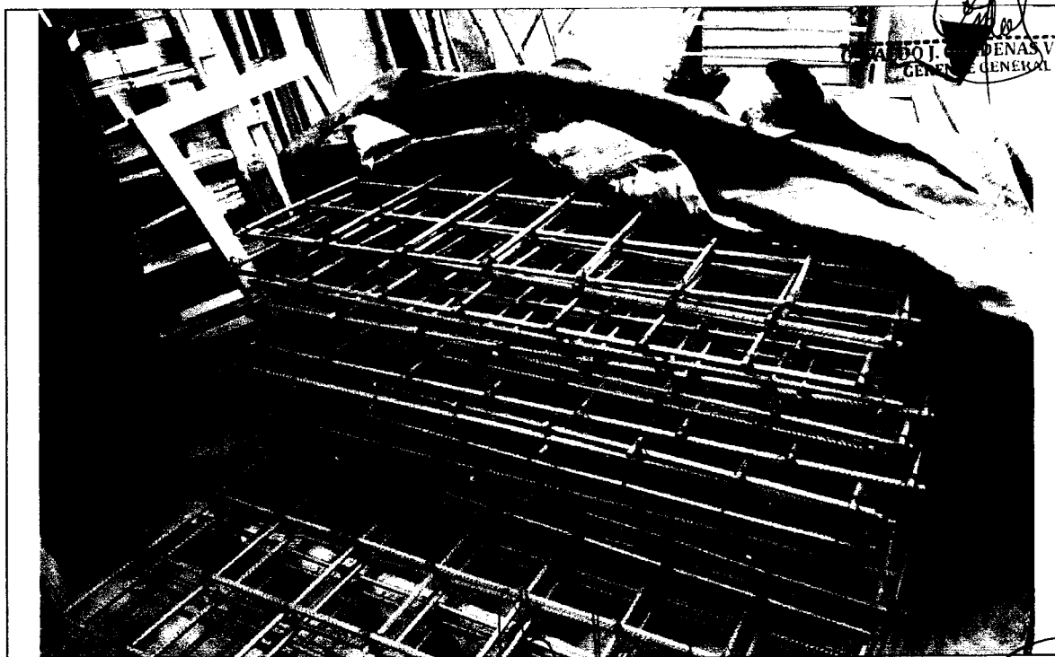
Foto N° 16: HABILITACION DE PARRILLAS PARA ZAPATAS.
